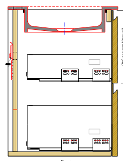
// Side SECTION
